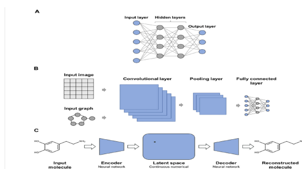
Рис 1. Пример продвинутых глубоких нейронных сетей. Показаны специализированные архитектуры DNN, включая (А) многозадачный DNN, (Б) сверточный DNN для обучения на основе молекулярных изображений или графов и (В) автоэнкодер в качестве примера архитектуры DNN для генеративного проектирования de novo.
